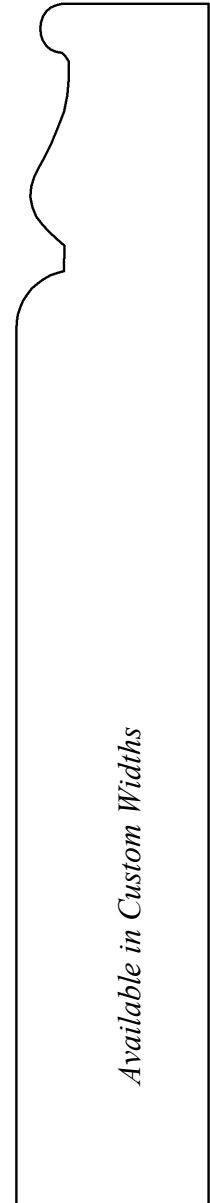
PB-100 1 1/4" X 6 1/4"
